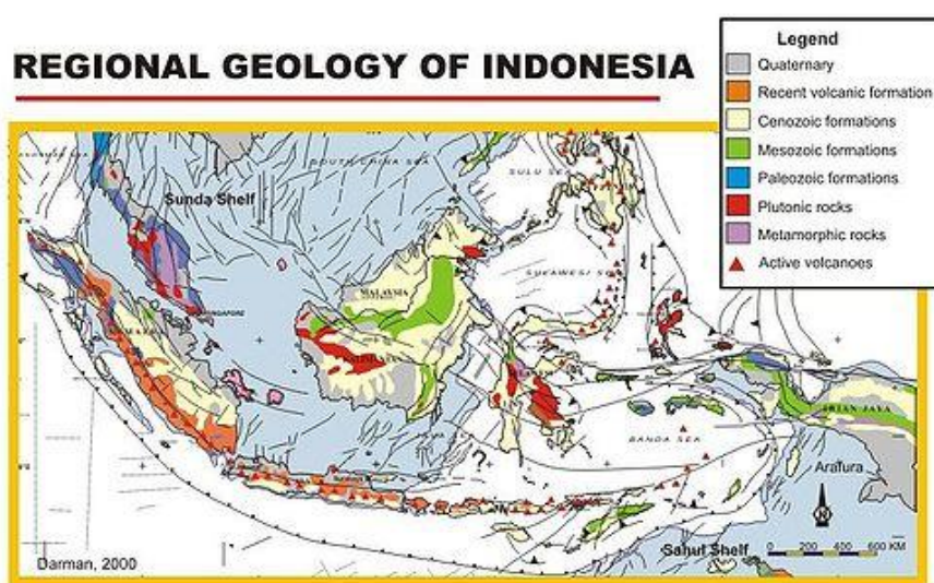
Rys.8. Budowa geologiczna Indonezji Źródło: http://de.wikipedia.org/wiki/Indonesien
